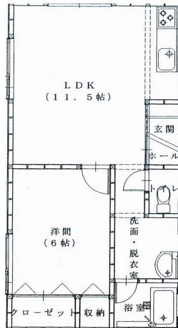
間取図
